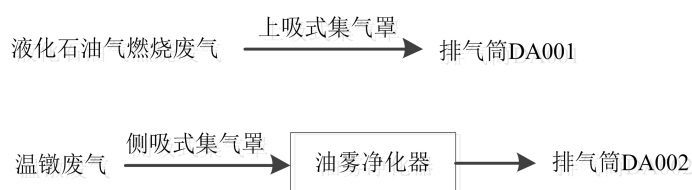
图 4-1 废气处理工艺流程
