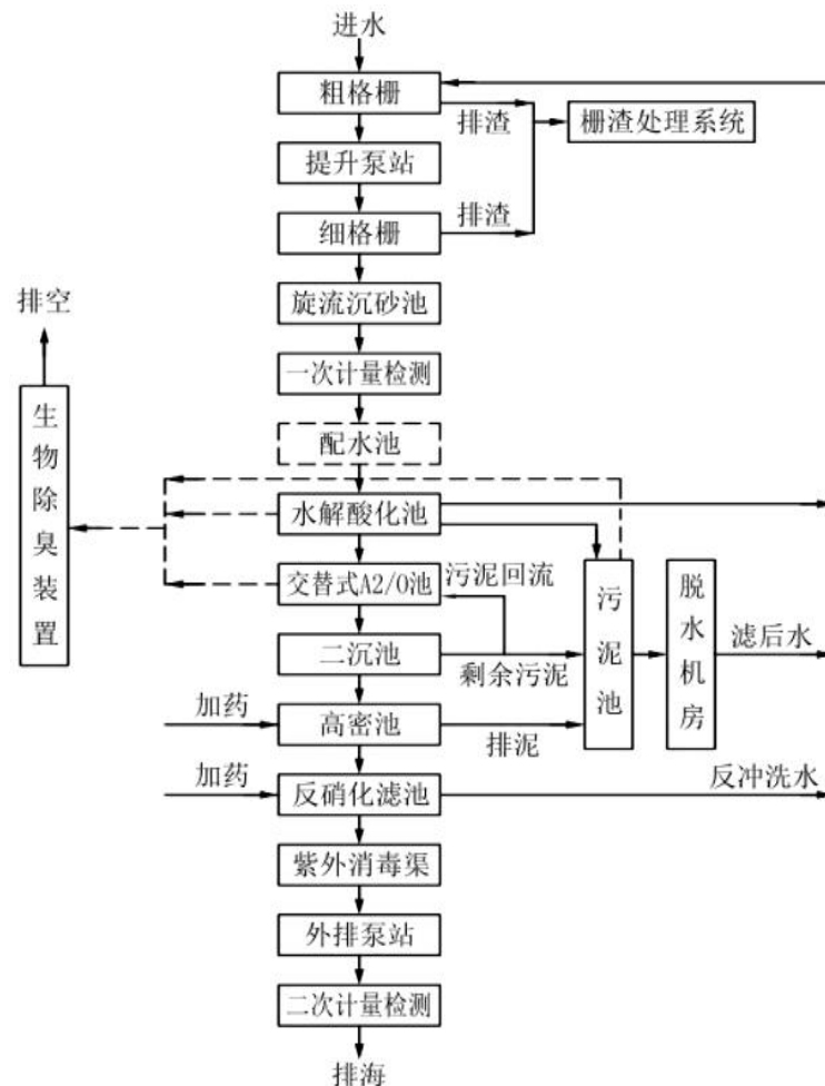
图 4-2 玉环市干江污水处理厂一期处理工艺流程图
