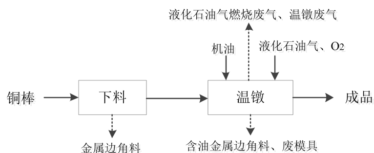
图 2-2 工艺流程图
